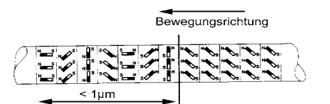
Abb. 3 Entmagnetisierungseffekt
