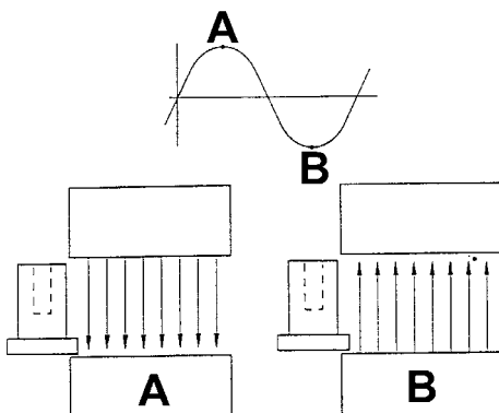
Abb. 5: Entmagnetisierungsdoppeljoch
