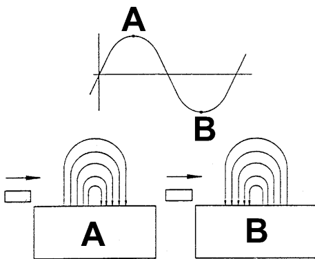
Abb. 4 Entmagnetisierungsjoch
